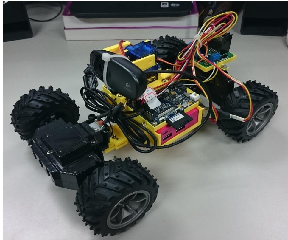
設計遙控車
