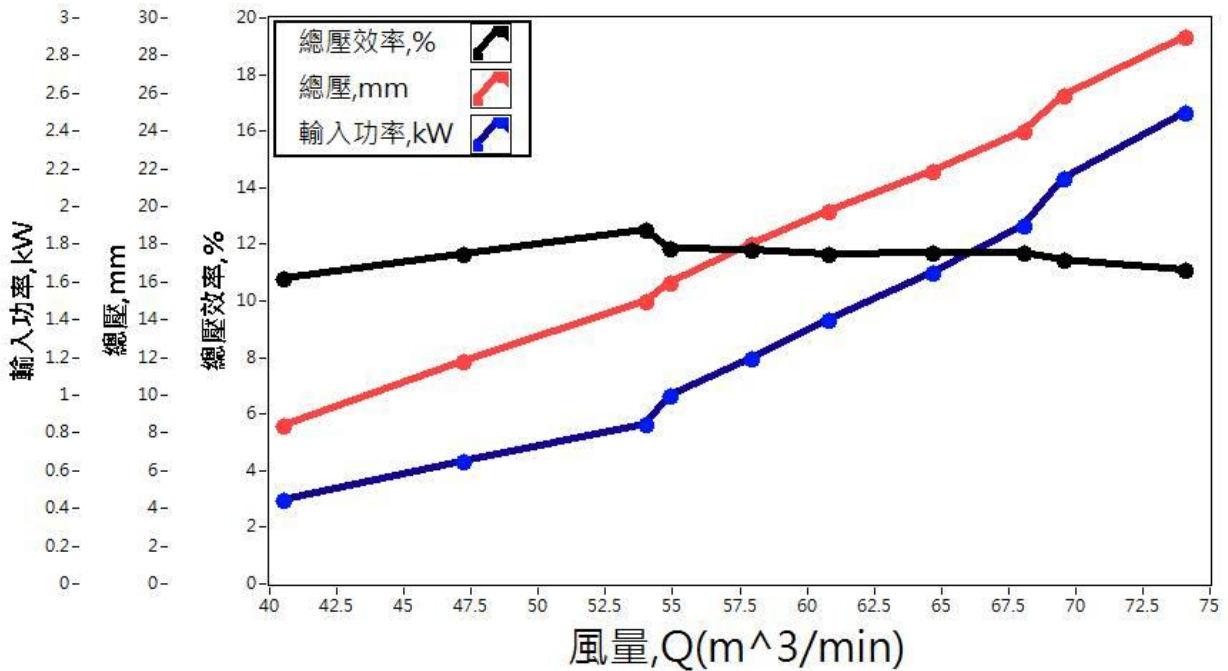
送風機性能圖
