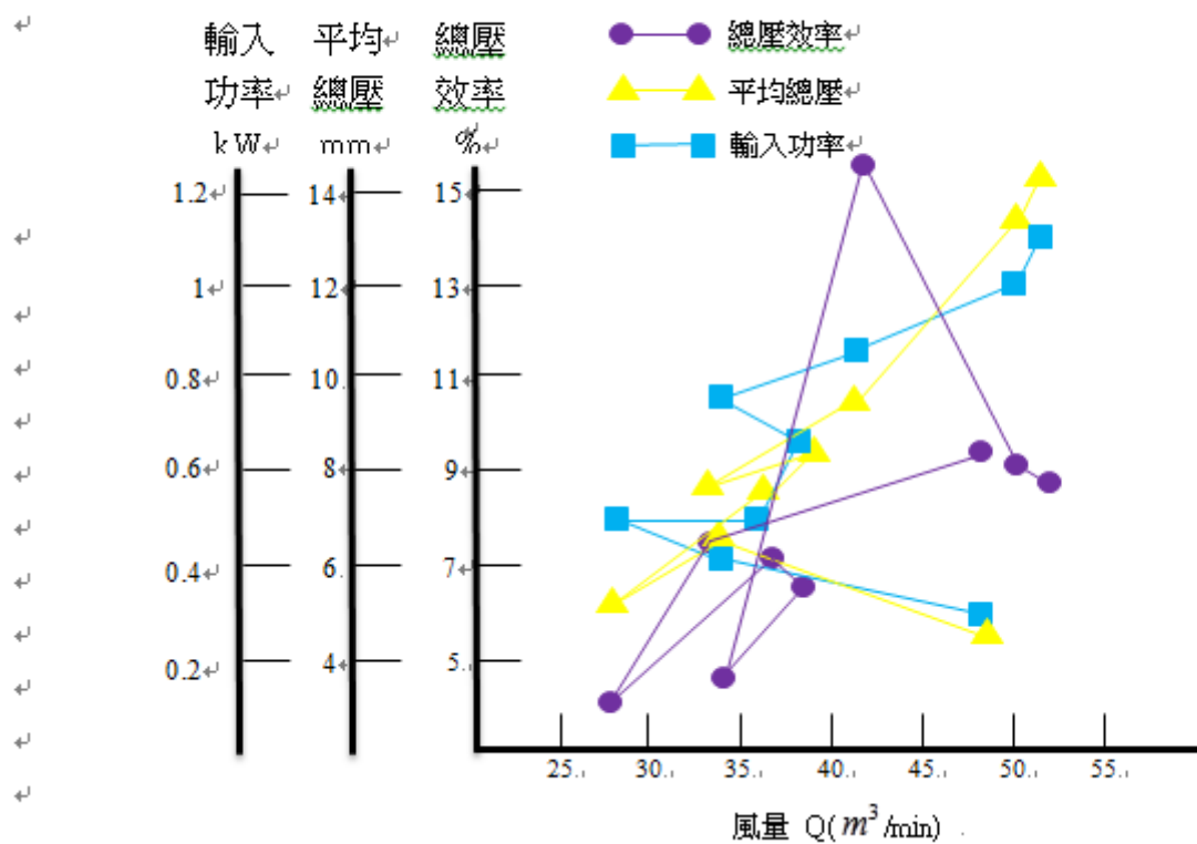
輸入功率，總壓，總壓效率 - 風量之變化圖
